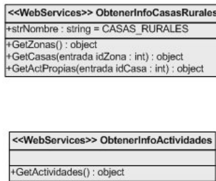
Figura 14.4. Diagrama de clases de servicios Web
