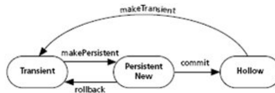
Figura 9.3. Estados correspondientes a la operación de hacer una instancia persistente.
