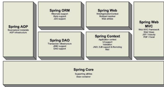
Figura 9.6. Arquitectura de Spring.
