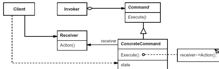
Figura 4.14. Estructura del patrón Command.
