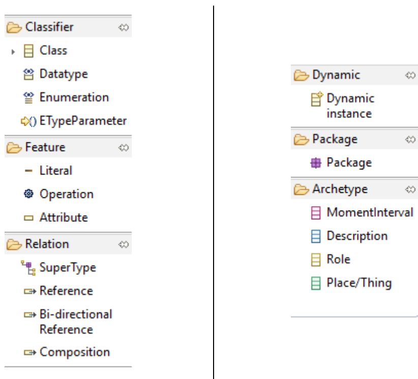
Ilustración 19 Sintaxis concreta gráfica de Ecore versión 2.11.2.v20160208-0816
