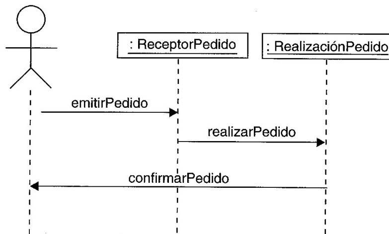
Diagrama de secuencia a un alto nivel de abstracción y poco detallado
