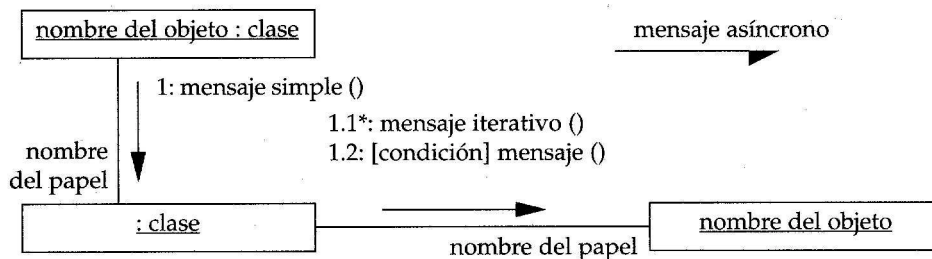
Diagrama de colaboración
