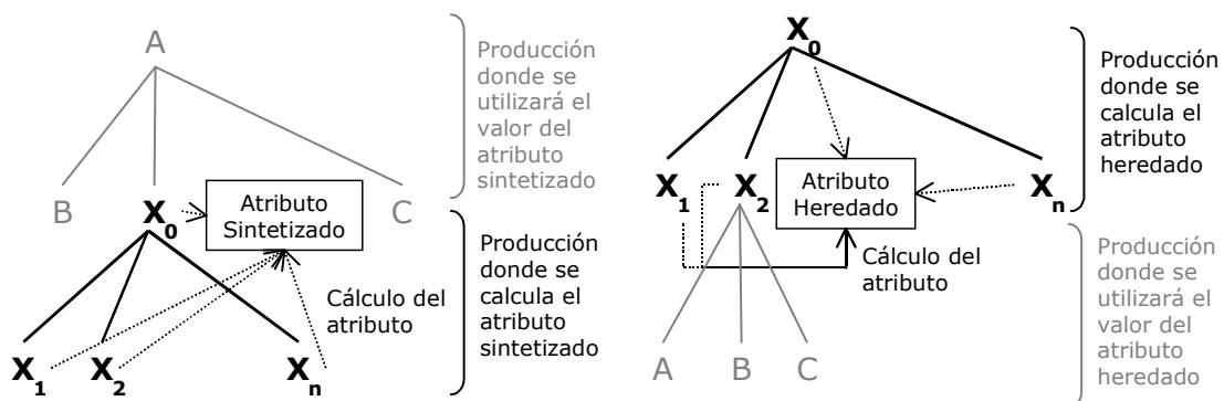
Figura 7: Evaluación de atributos heredados y sintetizados.
