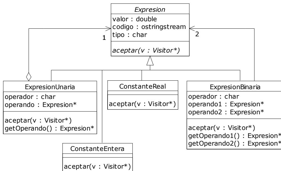
Figura 16: Estructura estática de los AST empleados para las expresiones del lenguaje presentado.
