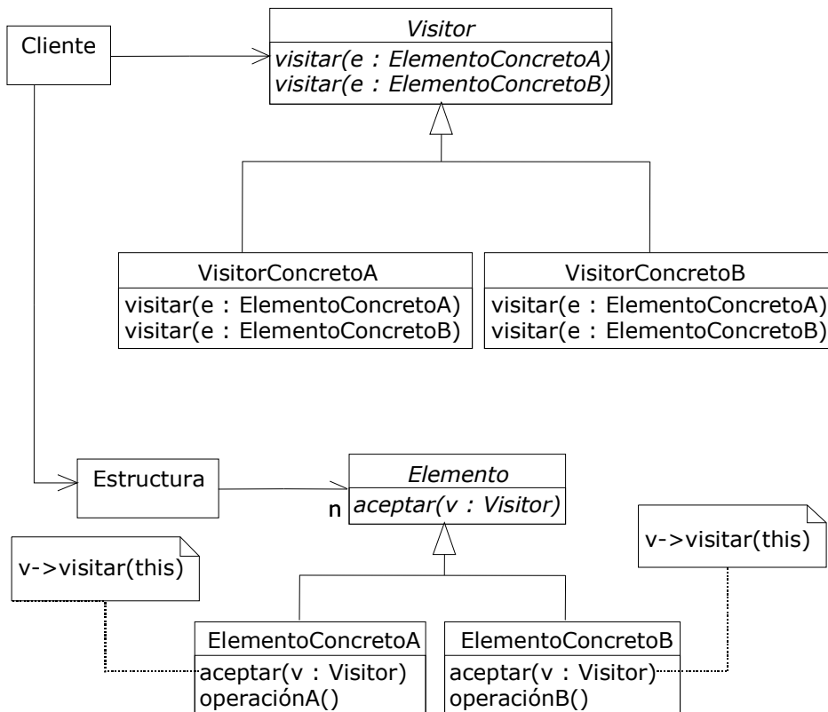
Figura 15: Diagrama de clases del patrón de diseño Visitor .
