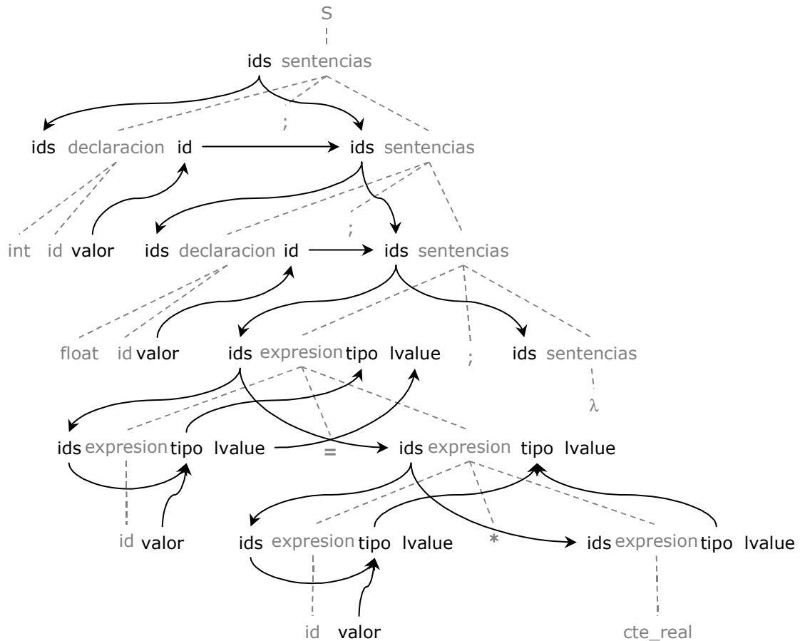
Figura 11: Grafo de dependencias para el cálculo de atributos, ante el programa especificado.
