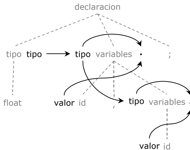
Figura 12: Grafo de dependencias para la entrada "float a,b;".
