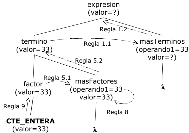
Figura 9: Árbol con anotaciones para el programa de entrada 33.
