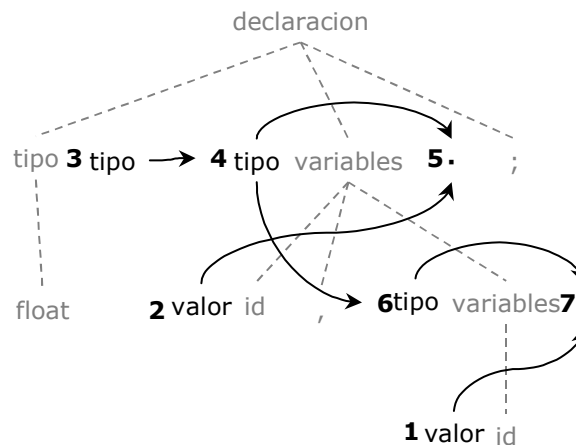
Figura 13: Numeración de los nodos del grafo de dependencias, estableciendo un ordenamiento topológico sobre el mismo.
