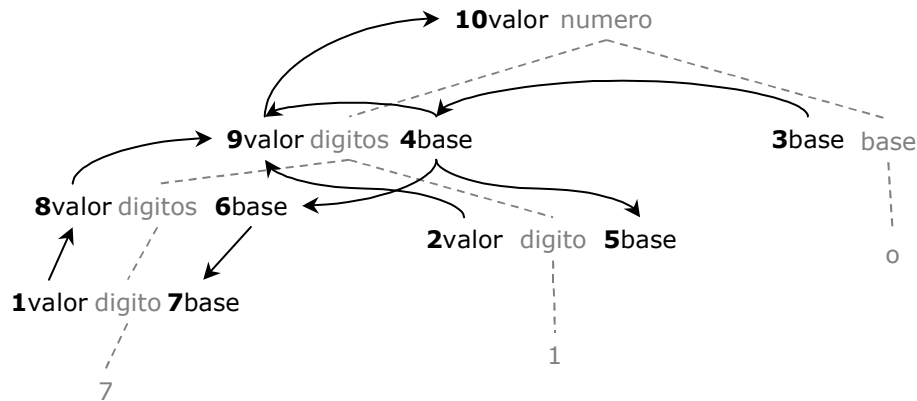
Figura 14: Grafo de dependencias para la entrada "710".
