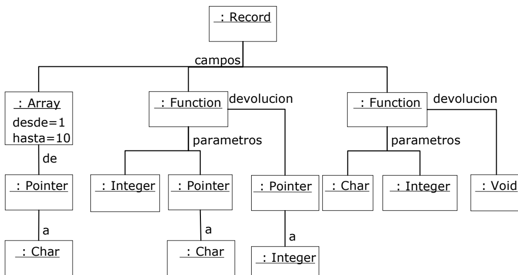
Figura 19: Diagrama de objetos creado a partir de la expresión de tipos especificada.
