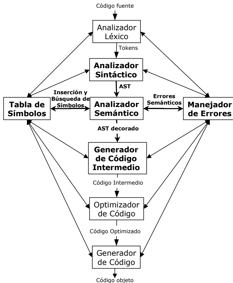
Figura 1: Fases de un compilador, destacando la interacción con el análisis semántico.
