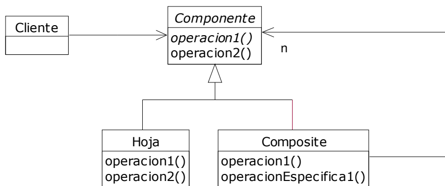
Figura 17: Diagrama de clases del patrón de diseño Composite .
