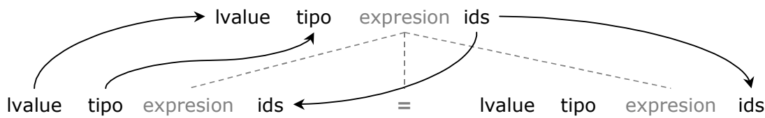
Figura 10: Grafo de dependencias locales para la producción que define las asignaciones.
