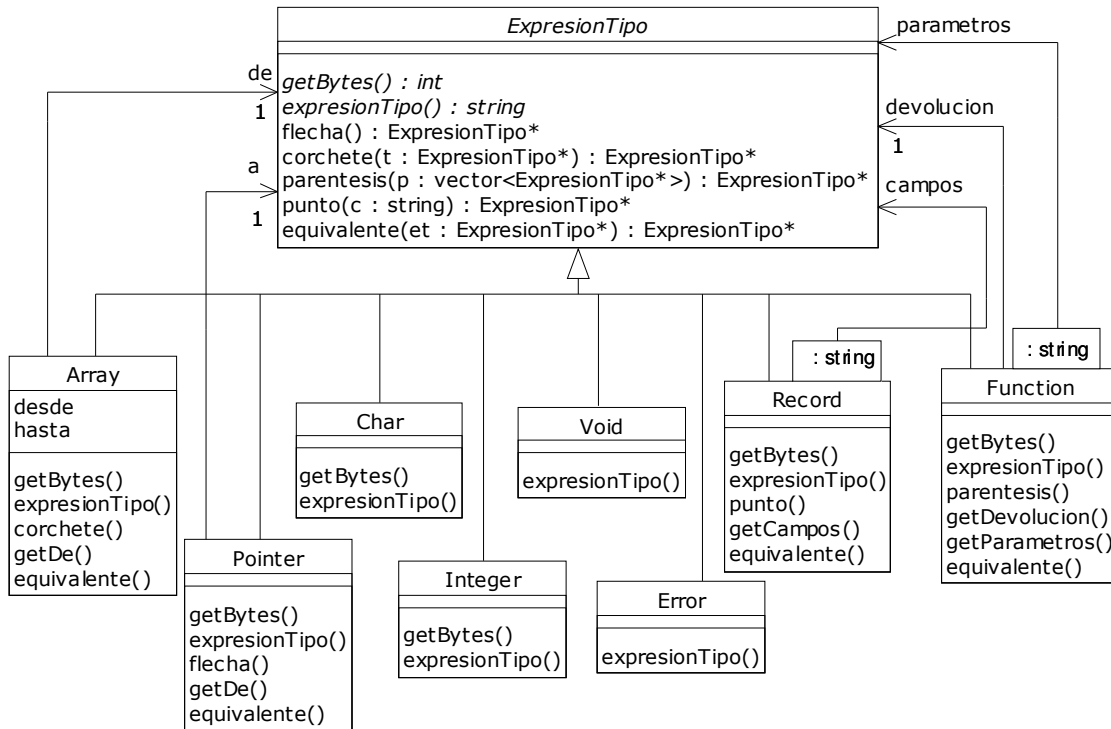
Figura 18: Diagrama de clases empleado para modelar expresiones de tipo.
